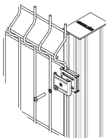
крепление «Скоба + Винт»
